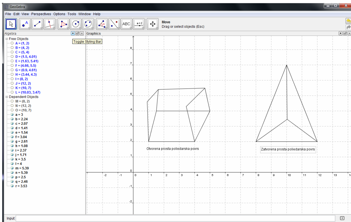
Slika 13. Konstrukcija otvorene i zatvorene proste poliedarske površi
