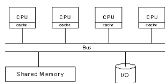
Симетрични мултипроцесор [23]
