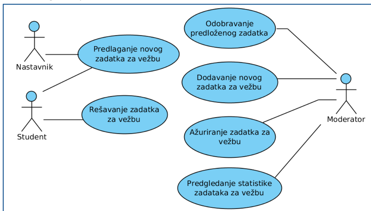
Slika 5b: Dijagram slučajeva upotrebe za modul vežbanje
