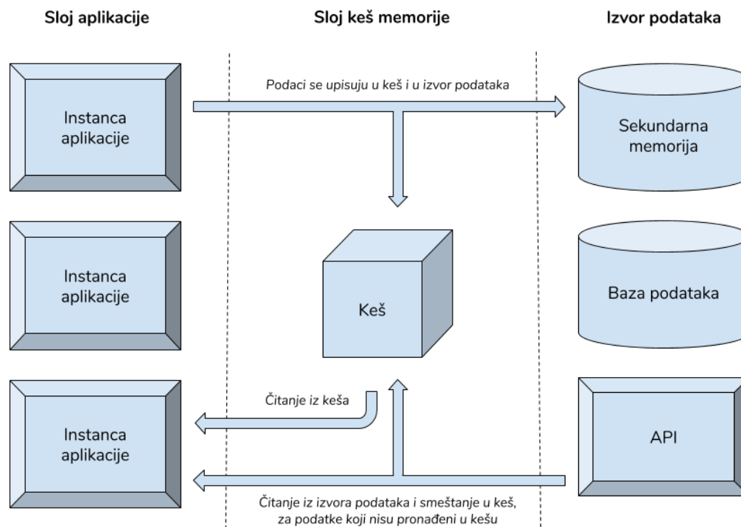
Slika 1.3 Arhitektura aplikacije koja koristi keš
