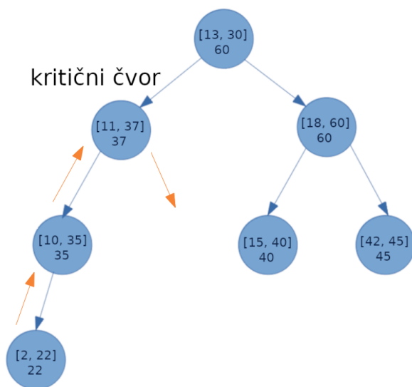
Slika 2.4: Intervalno stablo nakon umetanja novog intervala [2, 22]
