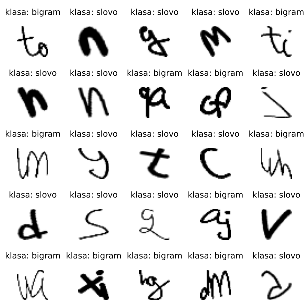
Slika 3.21: Test skup
