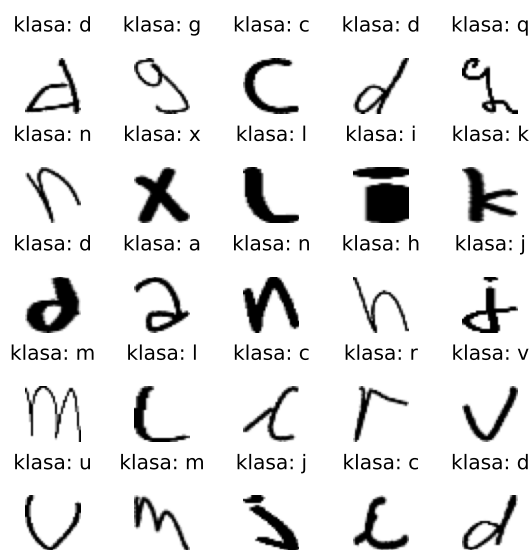
Slika 3.3: Test skup
