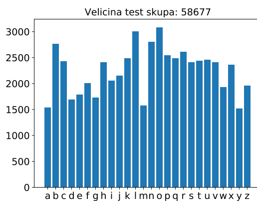
Slika 3.4: Raspodela podataka
