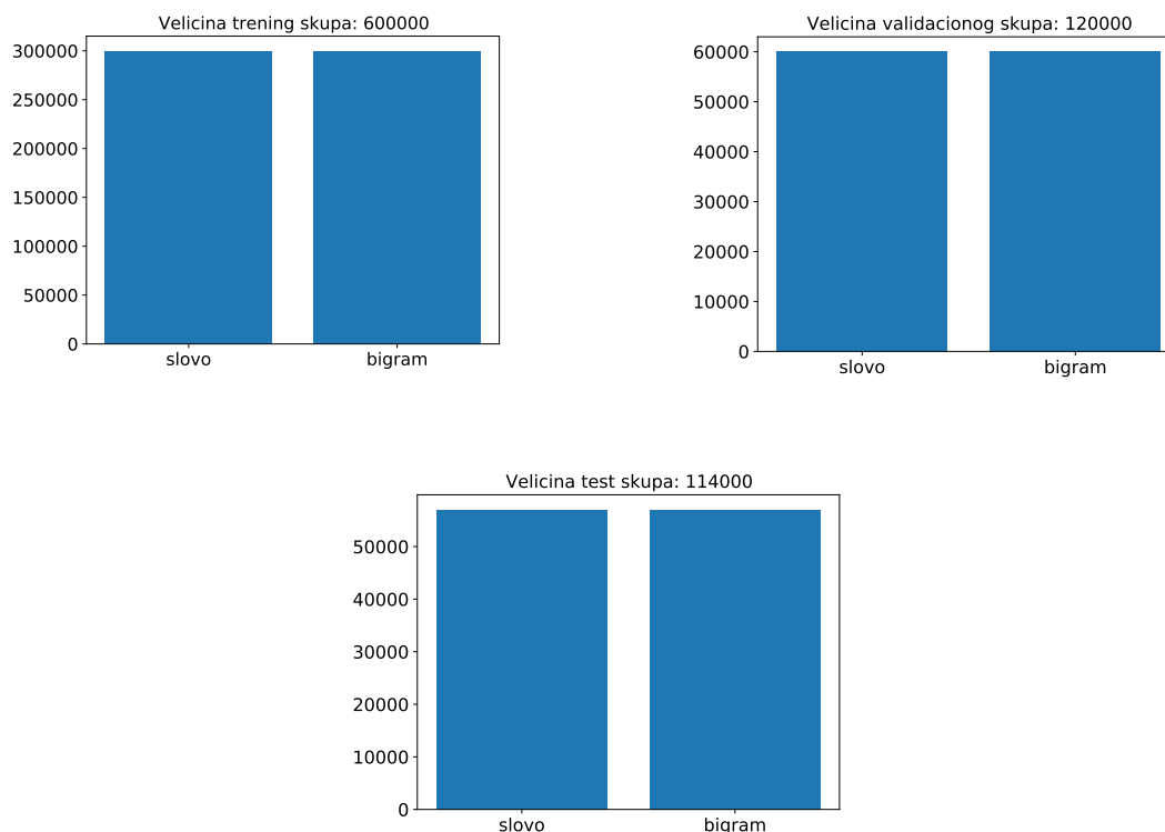
Slika 3.22: Raspodela podataka
