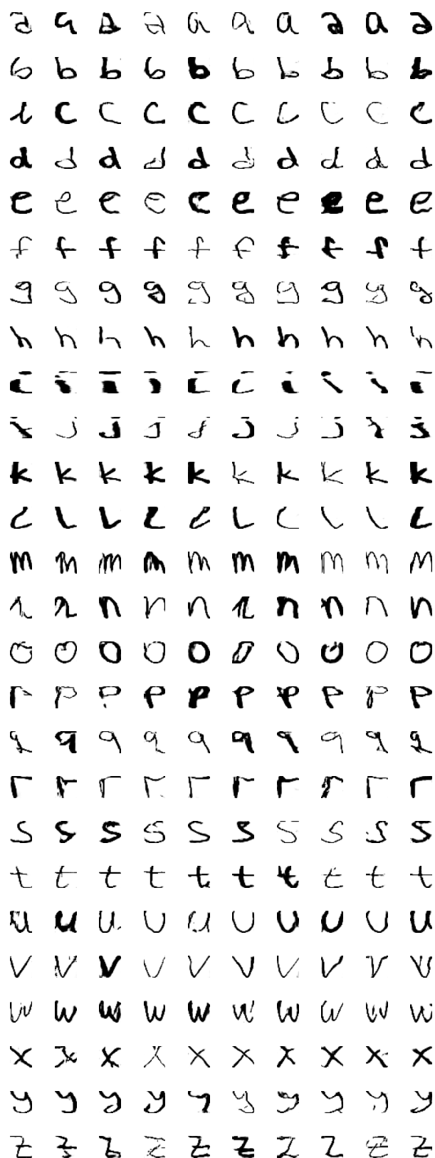
Slika 3.28: Generisani skup
