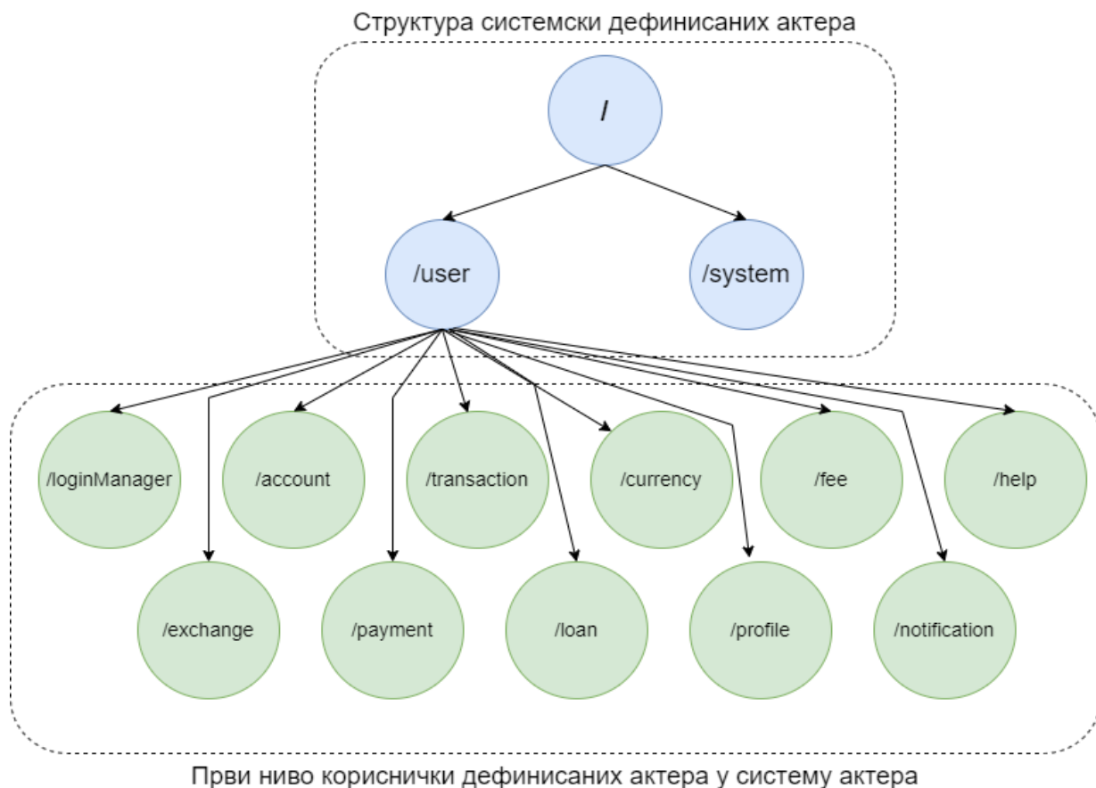
Слика 5.13 Приказ једне реплике система актера са првим нивоом актера дефинисаних од стране корисника
