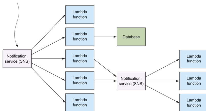
Slika 2.8: Primer upotrebe funkcije servisa AWS Lambda u projektnom uzorku grananje [preuzeto iz knjige Serverless architectures on AWS , autora Peter Sbarski, Yan Cui i Ajay Nair]
