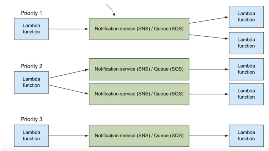
Slika 2.7: Primer upotrebe funkcije servisa AWS Lambda u projektnom uzorku sa prioritetskim nizovima
