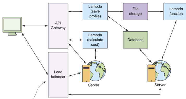
Slika 2.4: Primer upotrebe servisa AWS Lambda za kreiranje hibridnog rešenja [preuzeto iz knjige Serverless architectures on AWS , autora Peter Sbarski, Yan Cui i Ajay Nair]
