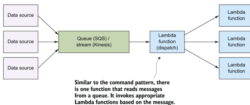
Slika 2.6: Primer upotrebe funkcije servisa AWS Lambda u projektnom uzorku sa porukama [preuzeto iz knjige Serverless architectures on AWS , autora Peter Sbarski, Yan Cui i Ajay Nair]
