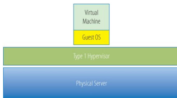
Slika 1.2: Hipervizor tip 1
