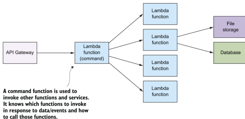
Slika 2.5: Primer upotrebe funkcije servisa AWS Lambda u Komanda projektnom uzorku
