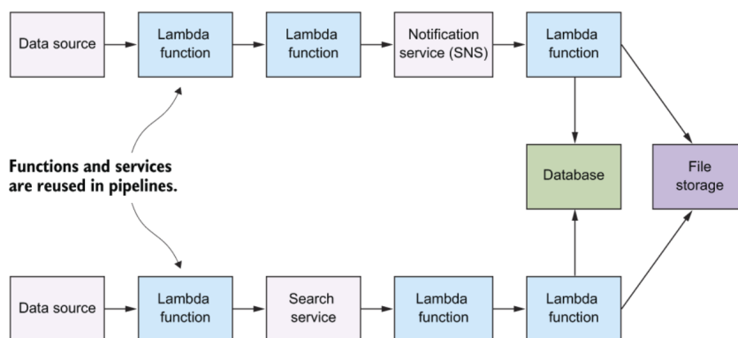
Slika 2.9: Primer upotrebe funkcije prilikom izrade kompleksnih sistema za obradu podataka [preuzeto iz knjige Serverless architectures on AWS , autora Peter Sbarski, Yan Cui i Ajay Nair]
