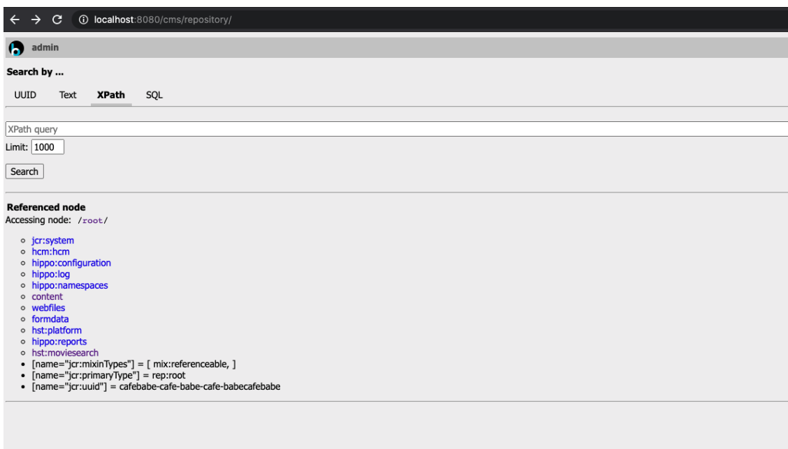
Slika 2.2: Repozitorijum
