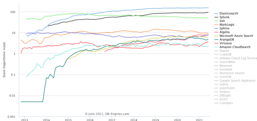
Slika 1.3: Elasticsearch popularnost
