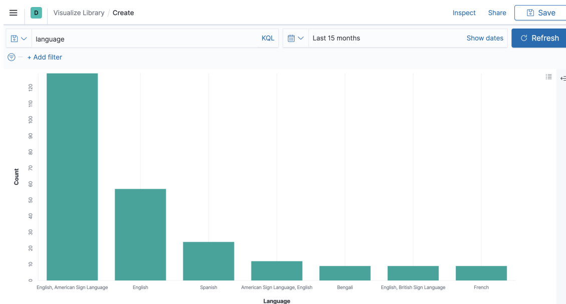
Slika 3.3: Kibana
