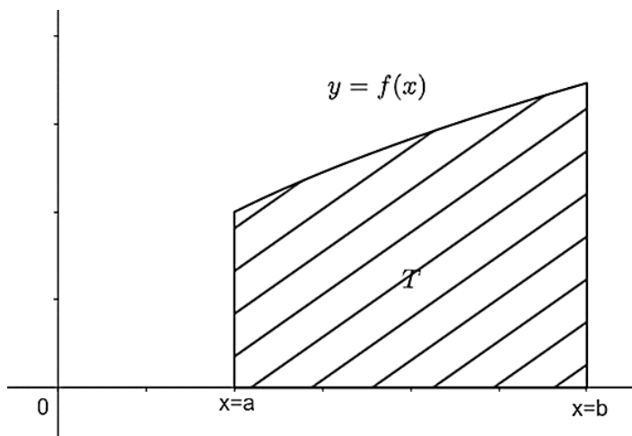
Слика 3.1. Површина криволинијског трапеза
