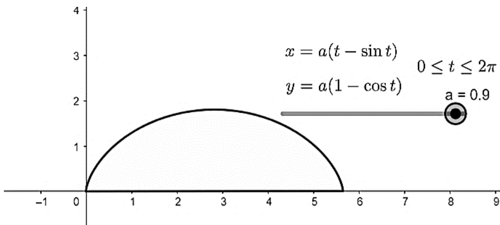
Слика 4.2.1. Дужина лука криве задате параметарски x = a(t - \sin t);
